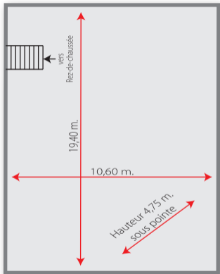
ÉTAGE
